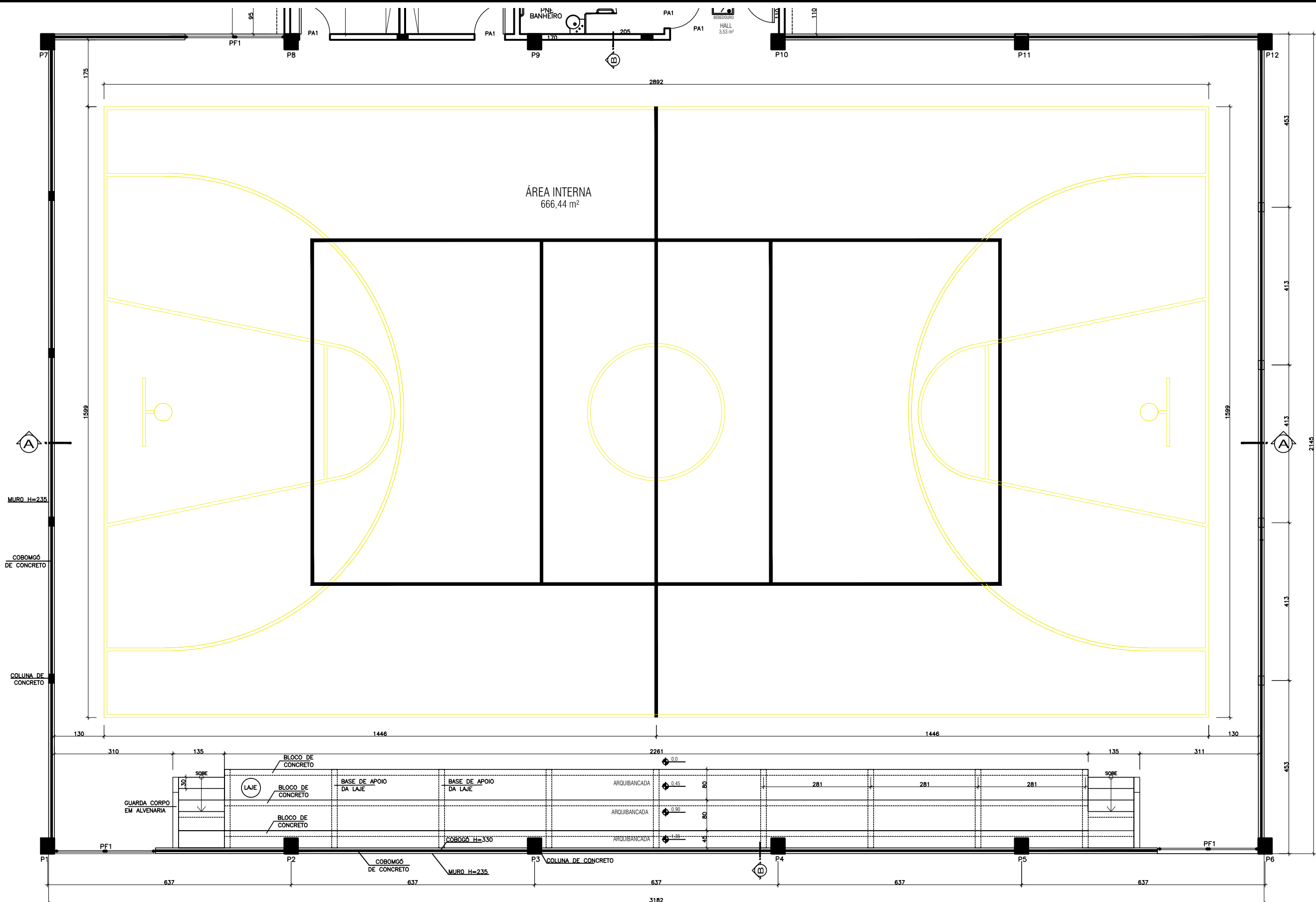
PLANTA QUADRA
